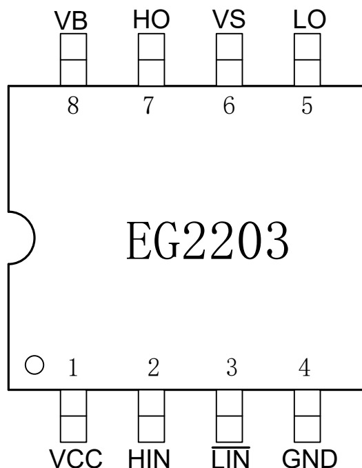
图 4-1. EG2203 管脚定义
