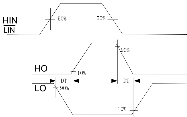
图 7-1. 低端输出 LO 开关时间波形图
