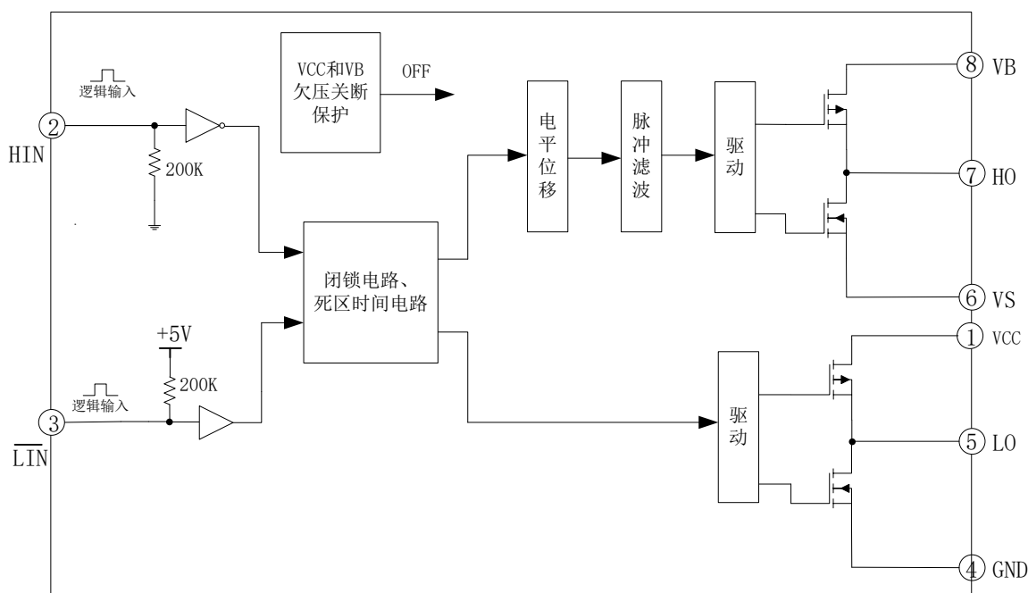
图 5-1. EG2203 内部电路图
