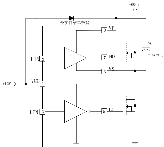
图 8-3. EG2203 自举电路结构
