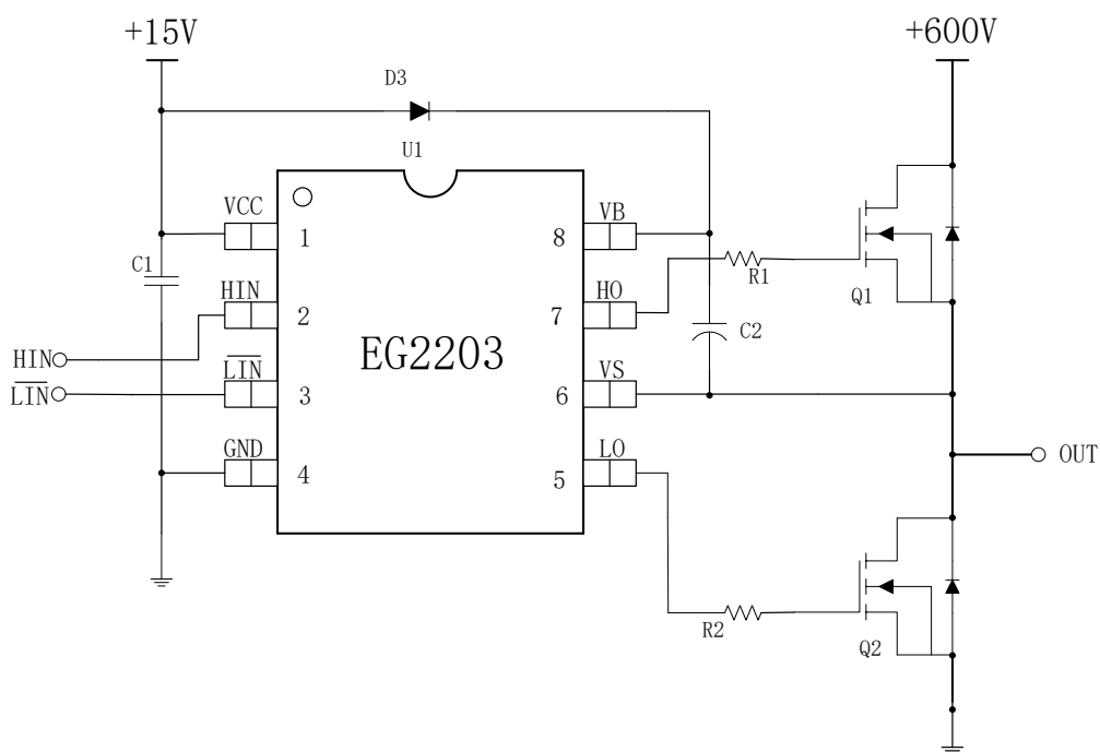
图 6-1. EG2203 典型应用电路图
